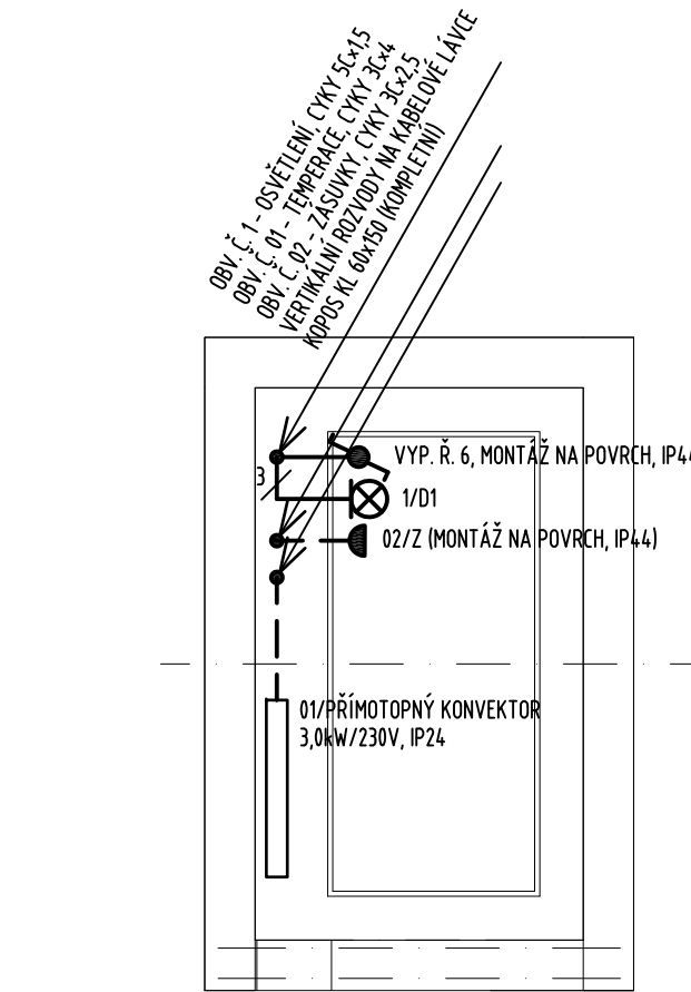
PODLAŽÍ 1.NP
