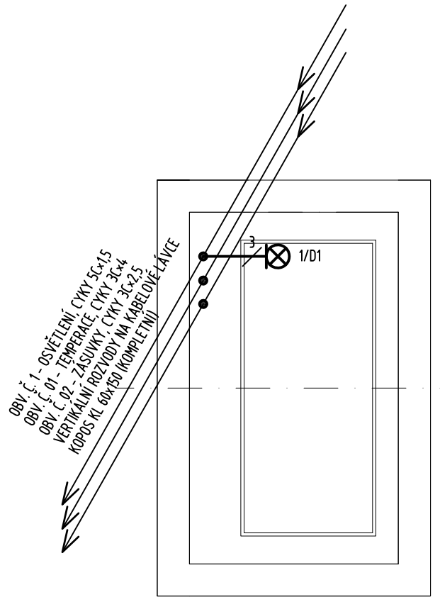
PODLAŽÍ 2.NP
