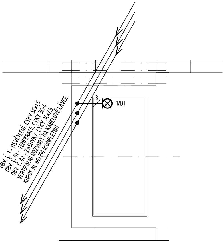
PODLAŽÍ 3.NP
