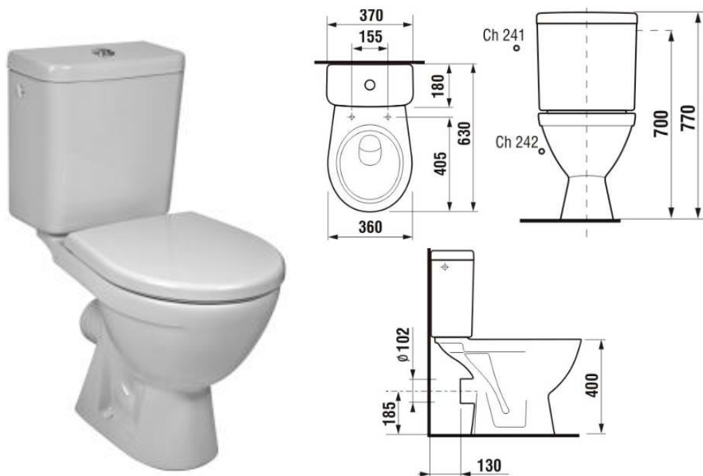
Obrázek 3 – vzhled a technický výkres klozetu JIKA LYRA PLUS WC kombi - vodorovný odpad
